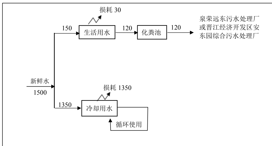
图 2.7-1 项目水平衡图(t/a)
