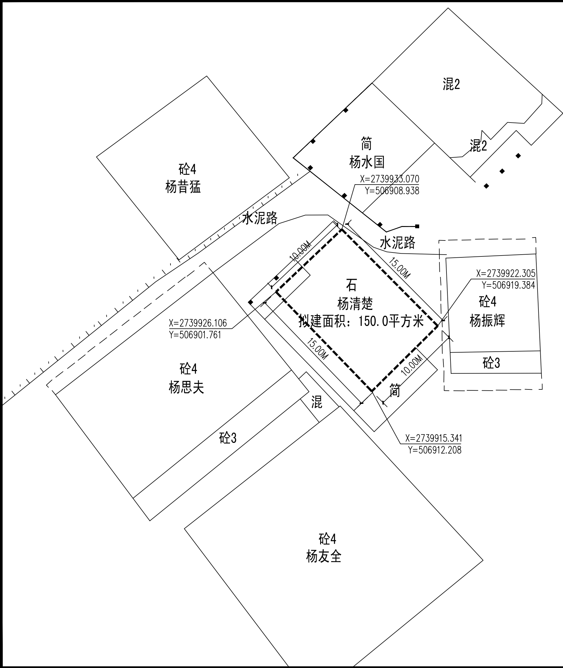
总平面图1:250
