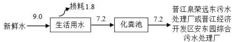
图 2-1 项目水平衡图 (t/d)
