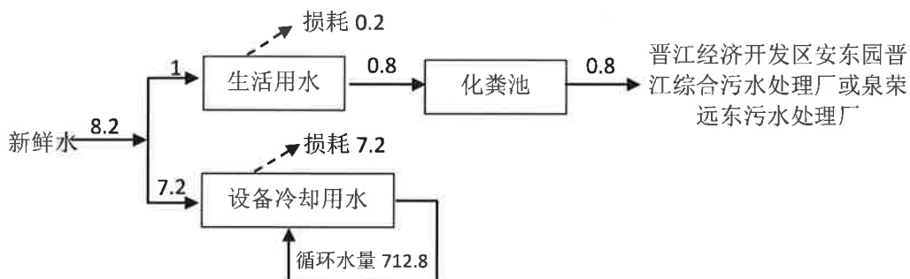
图 2.7-1 项目水平衡图 (t/d)
