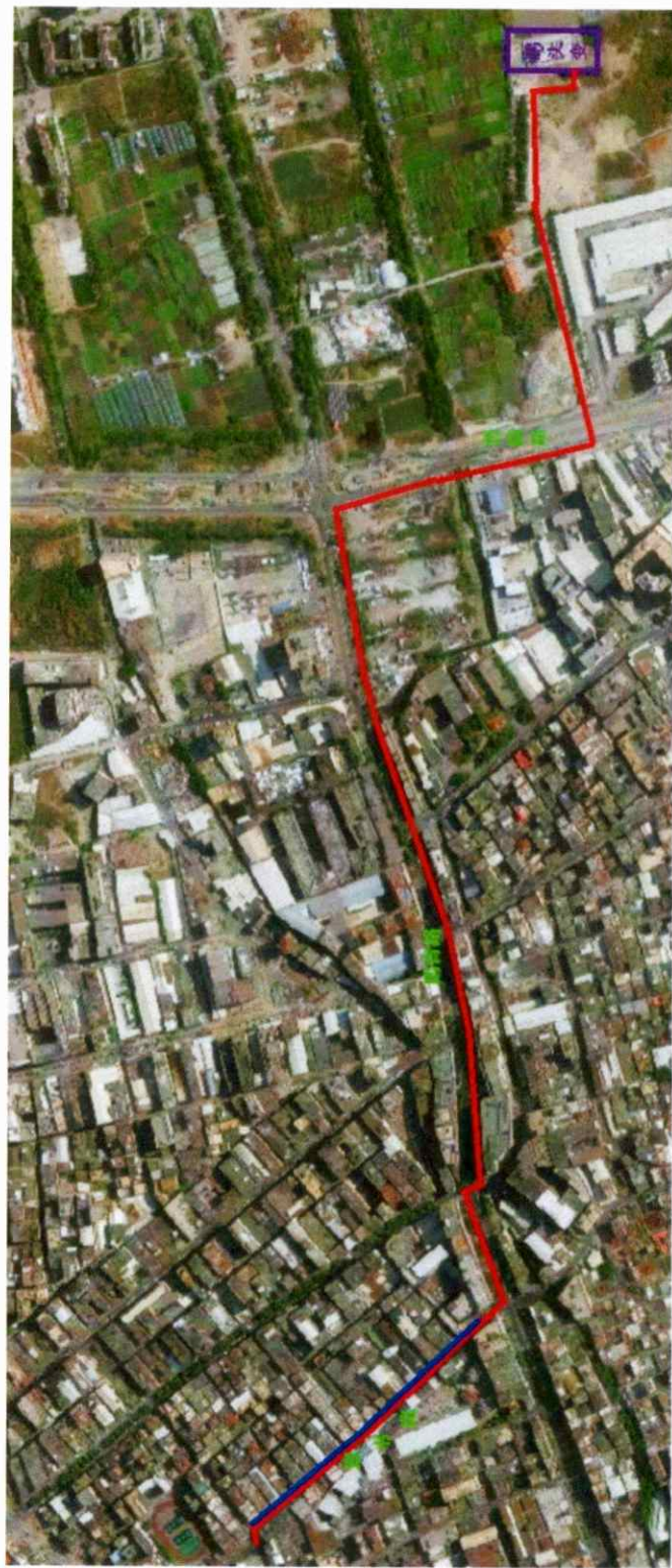
4.10 千伏聚书线电力线路路径简图
