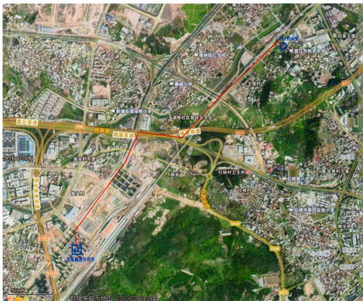
2.10 千伏西苑Ⅱ回电力线路路径简图
