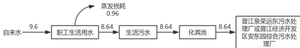
图2-1 项目水平衡图 单位：t/d
