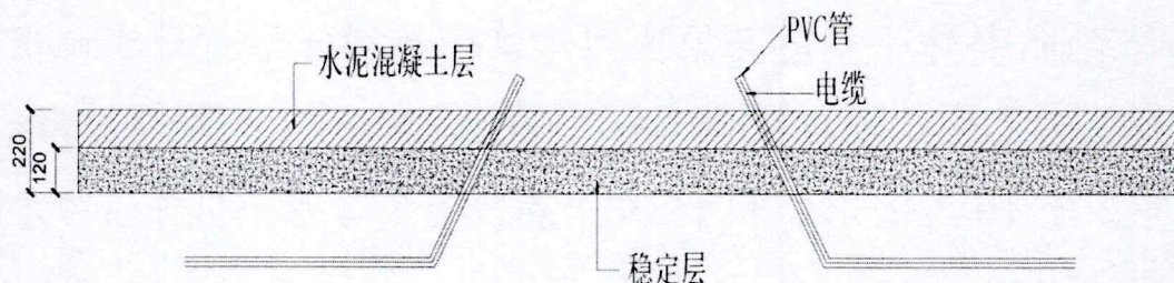
灯柱位置施工图
