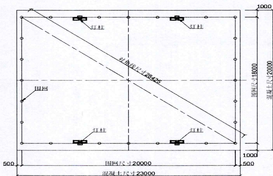
场地基础施工 及测量方法
