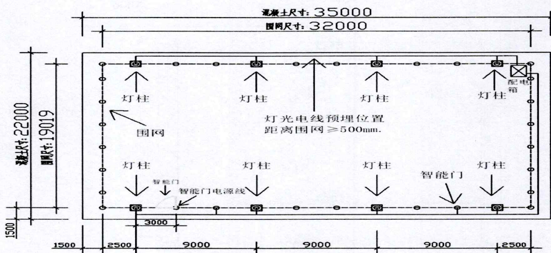
电缆及 PVC 管走线图
