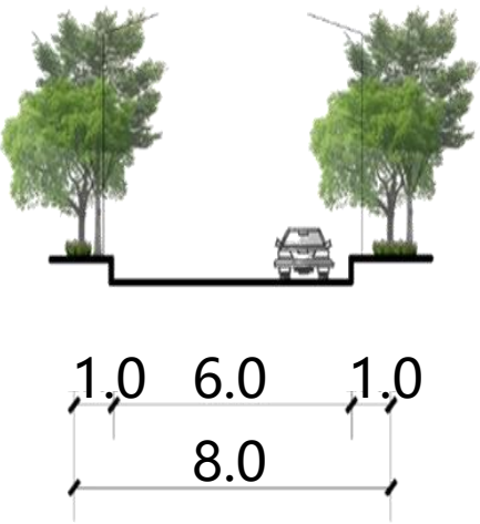
C-C道路断面图
