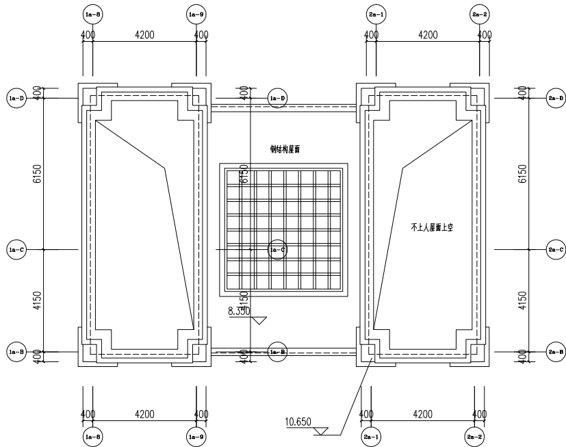
大门修改后屋顶局部平面图
