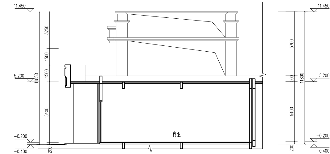
大门东修改前立面图
