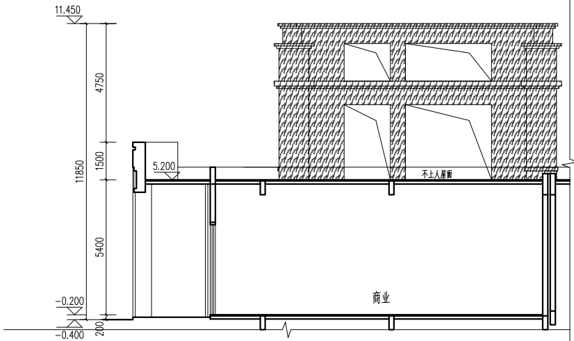
大门东修改后立面图
