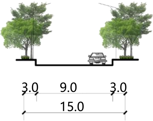
B-B道路断面图
