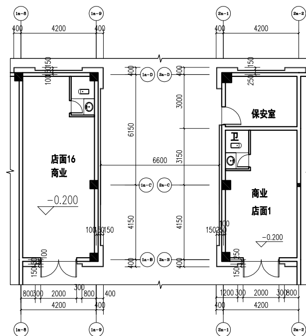
大门修改后一层局部平面图
