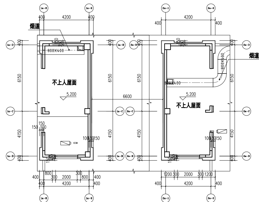
大门修改后屋面层局部平面图
