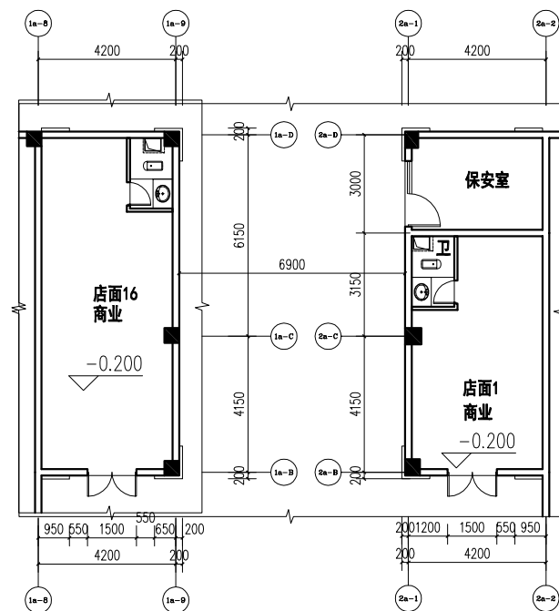
大门修改前一层局部平面图
