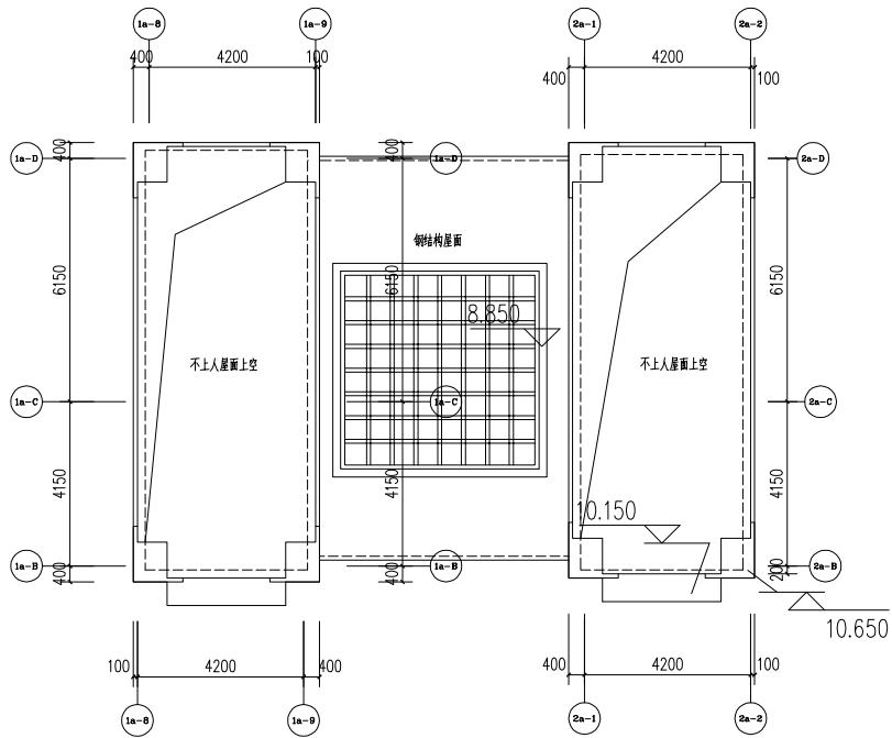
大门修改前屋顶局部平面图
