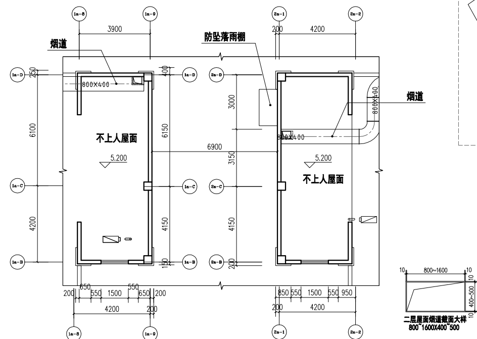
大门修改前屋面层局部平面图
