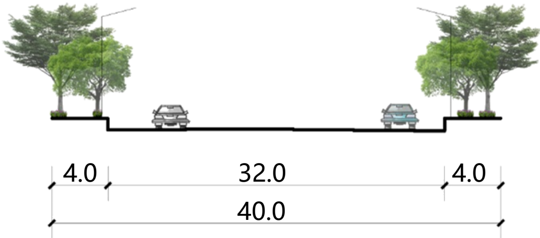
A-A道路断面图
