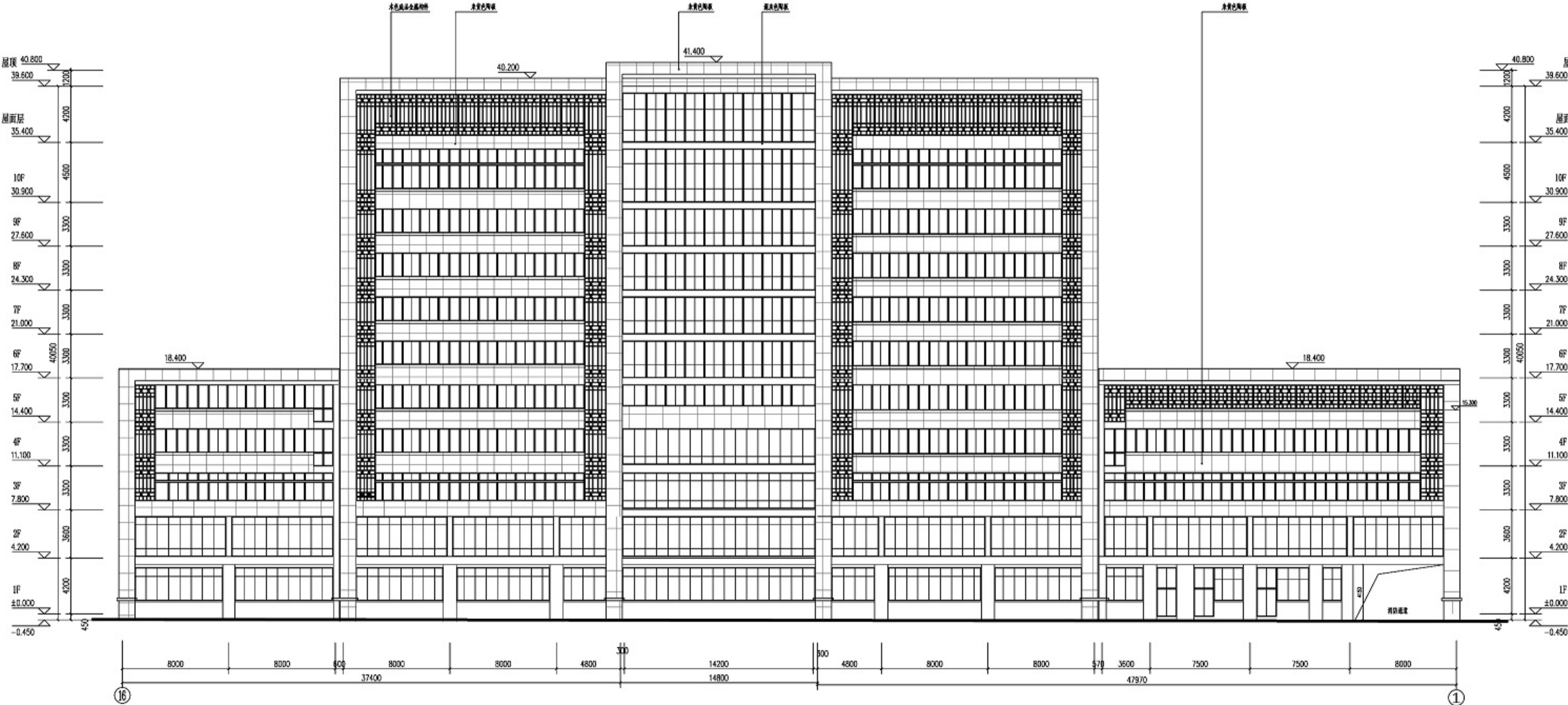
⑩ ~ ① 轴沿街立面展开图 (调整前)
