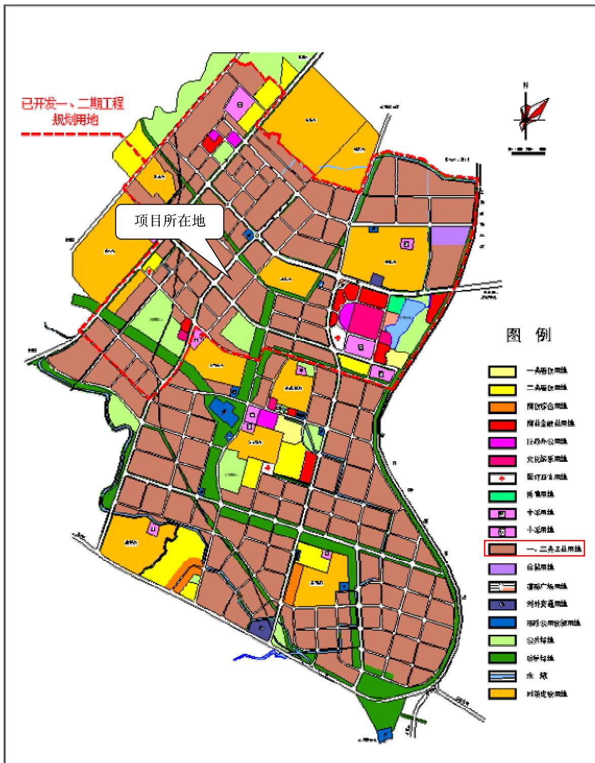
附图 8 晋江经济开发区（五里园）控制性详细规划修编-土地利用规划图
